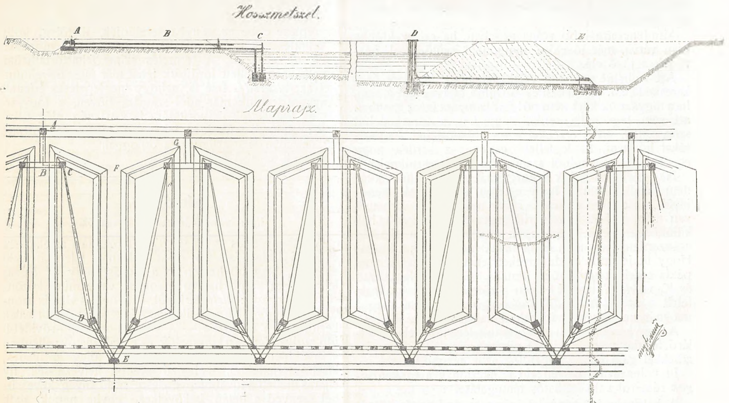
1. kép. Telető medenczék elrendezése.
