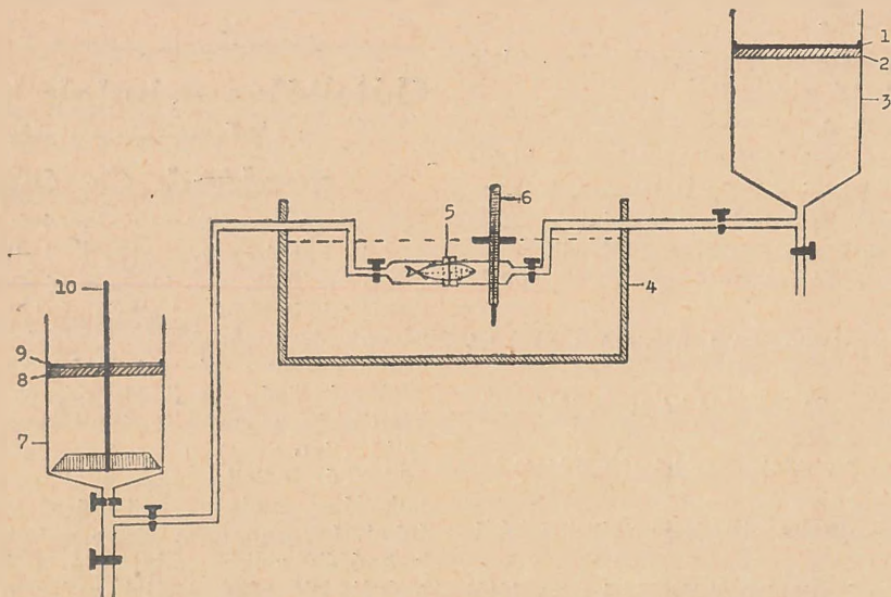
3. sz. ábra. 1 — alumíniumlemez, 2 — paraffinolaj réteg, 3 — felső víztartály, 4 — vízfürdő, 5 — edény a kísérleti állat befogadására, 6 — hőmérő a hőmérséklet ellenőrzésére, 7 — alsó víztartály, 8 — paraffinolaj réteg, 9 — alumíniumlemez, 10 — keverő.
